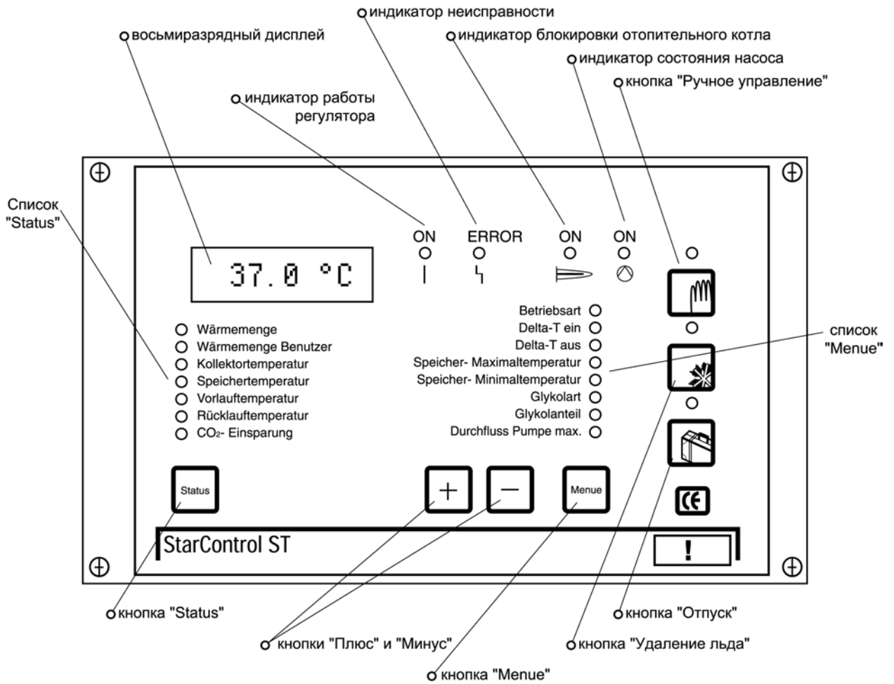
Рис. 1. Передняя панель регулятора Wilo-StarControl STE
