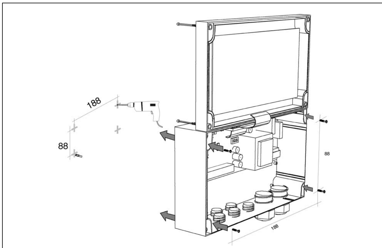
Рис.4.1. Монтаж корпуса
