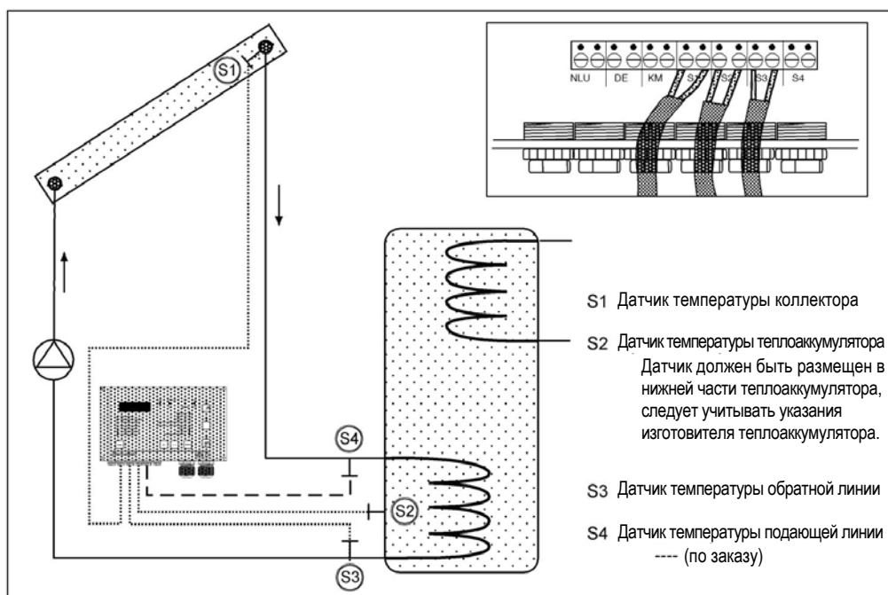
Рис.4.2 Установка и подключение датчиков температуры
