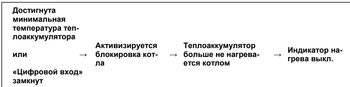
Рис.6.2 Блокировка нагрева
