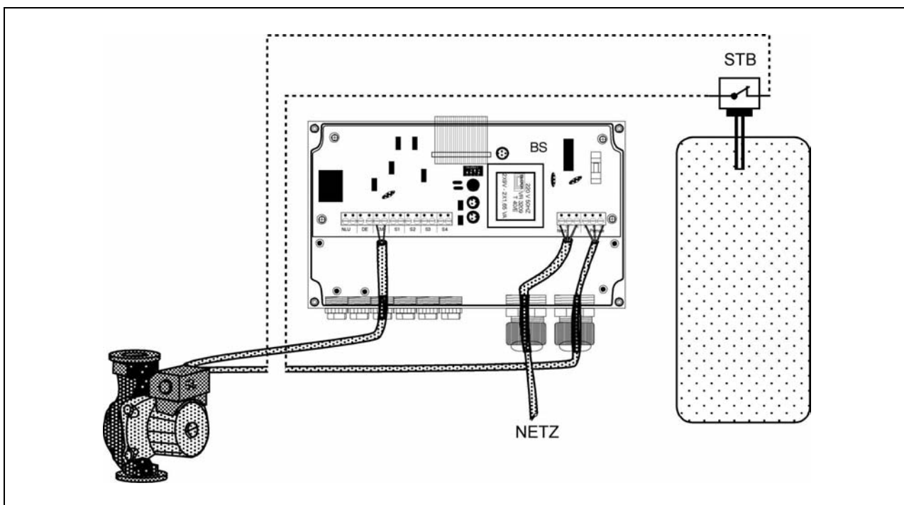
Рис.6.3. Система с предохранителем по температуре
