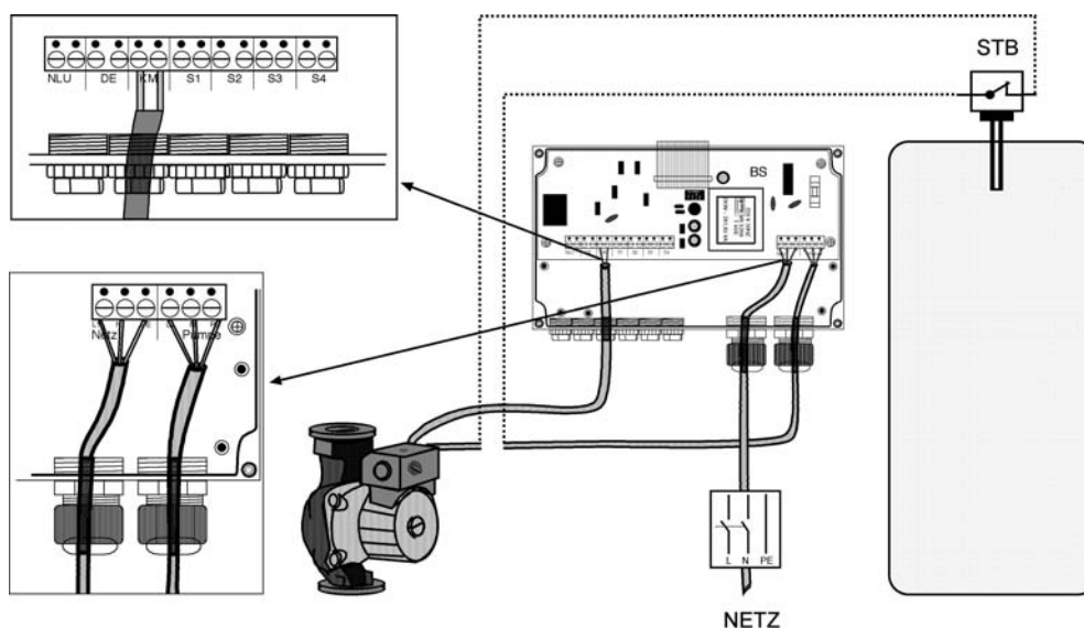
Рис.4.3 Подключение насоса, STB и кабеля питания от электросети
