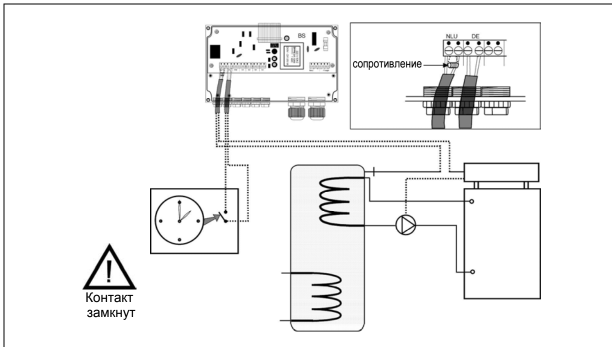
Рис. 4.4 Блокировка нагрева теплоаккумулятора котлом
