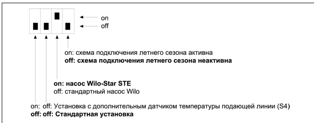
Рис.4.5 Джамперный переключатель с заводской настройкой
