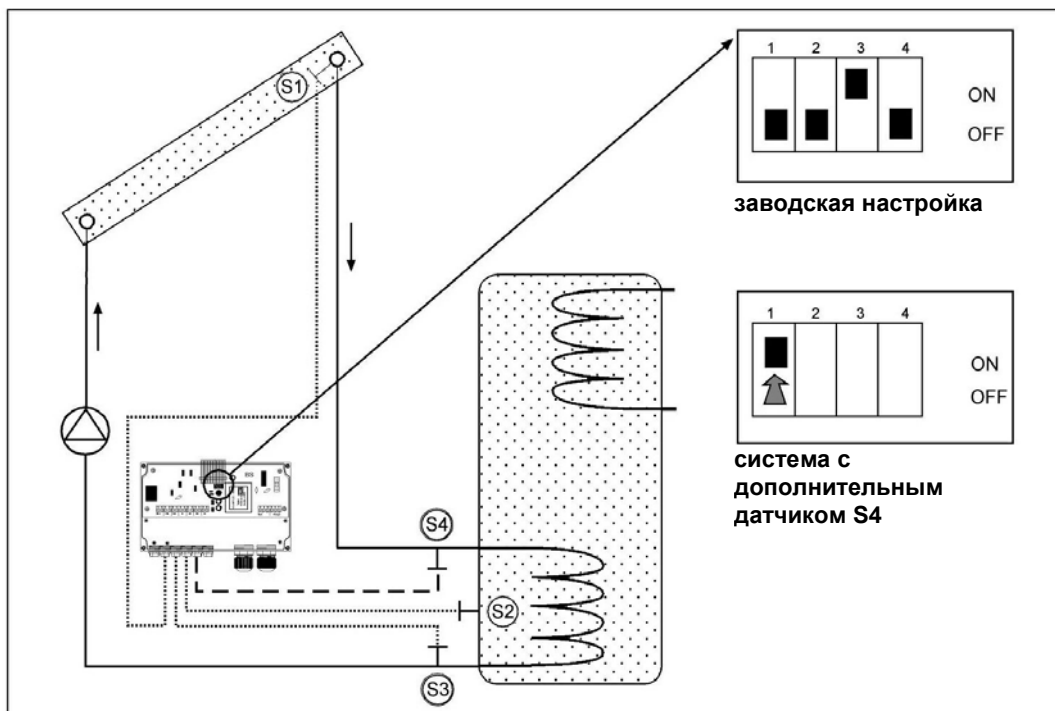
Рис. 6.1. Схема установки, настройка джамперного переключателя
